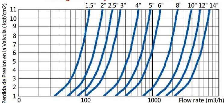
Diafragma de Flujo de Valvula Flotadora
