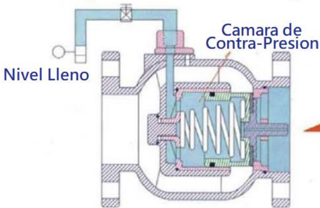
[Valvula en estado Cerrado]
