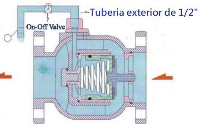
[Valvula en estado Abierto]
